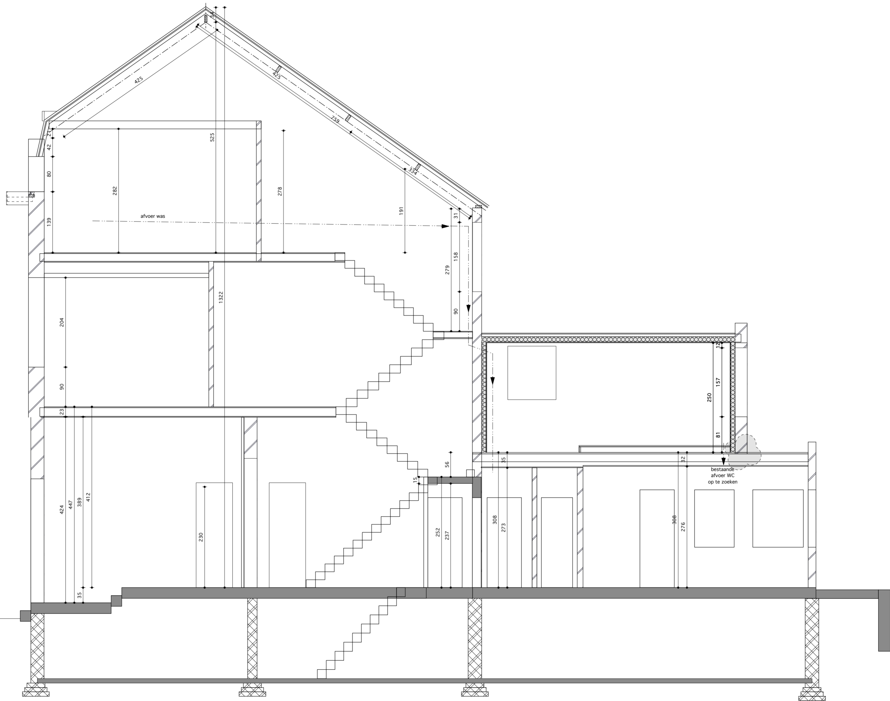
DOORSNEDE AA nieuwe toestand schaal 1/50
